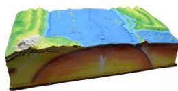
Modelo Formación De La Tierra
